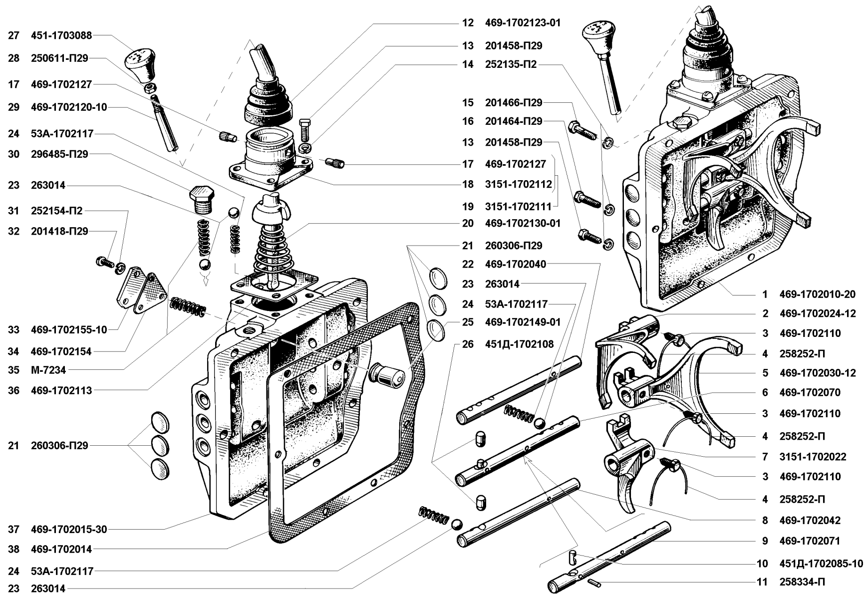
Рис. 46. Механизм переключения передач (1702)
